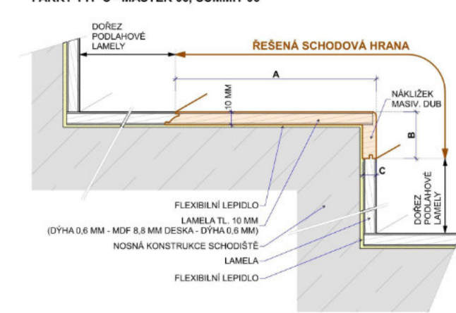
PARKY TYP C - MASTER 06, SUMMIT 06
