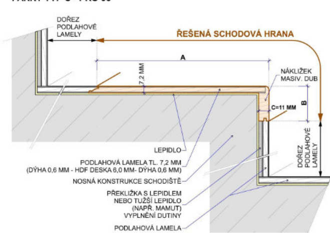
PARKY TYP C - PRO 06
